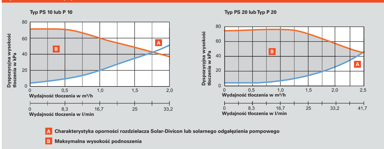
Rys. B.3.1-10 Charakterystyki Solar-Divicon
