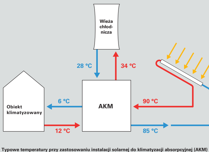
Rys. C.2.5-2 Temperatury przy zastosowaniu klimatyzacji Absorpcyjnej
