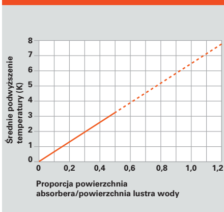
Rys. C.2.4-2 Podwyższenie temperatury w basenie otwartym
