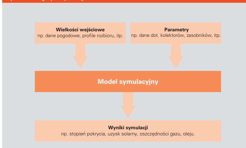
Rys. C.4-1 Algorytm symulacji
