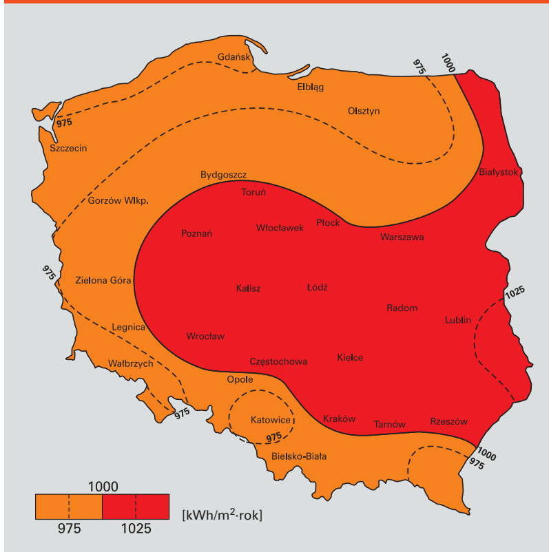
Rys. A.1.2-4 Promieniowanie całkowite w Polsce
