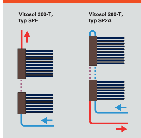
Rys. C.1.1-5 Warianty pionowego połączenia kolektorów (Vitosol 200-T)
