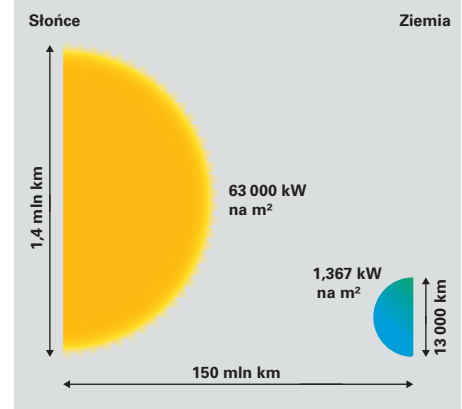
Rys. A.1.1-2 Stosunek Słońca do Ziemi
