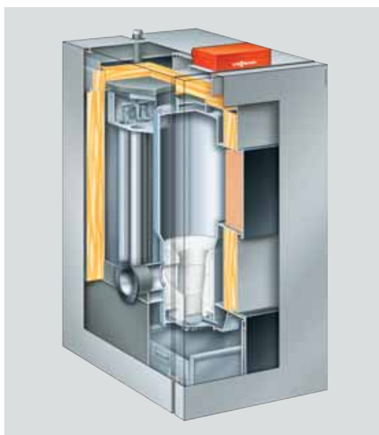
Fot. C.3.1-1 Vitoligno 300-P Kocioł na pelet
