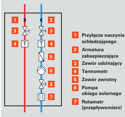
Rys. B.3.1-8 Schemat Solar-Divicon
