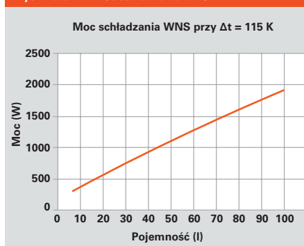
Rys. B.3.5-7 Moc schładzania WNS
