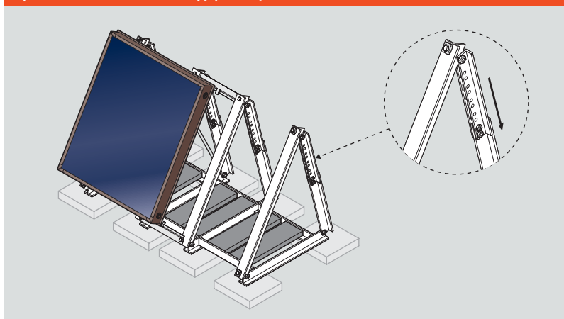
Rys. B.1.6–10 Montaż wolnostojący z obciążeniami
